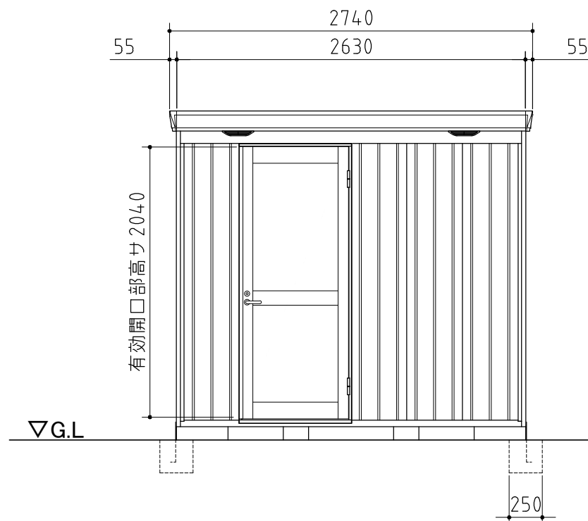
正面図
